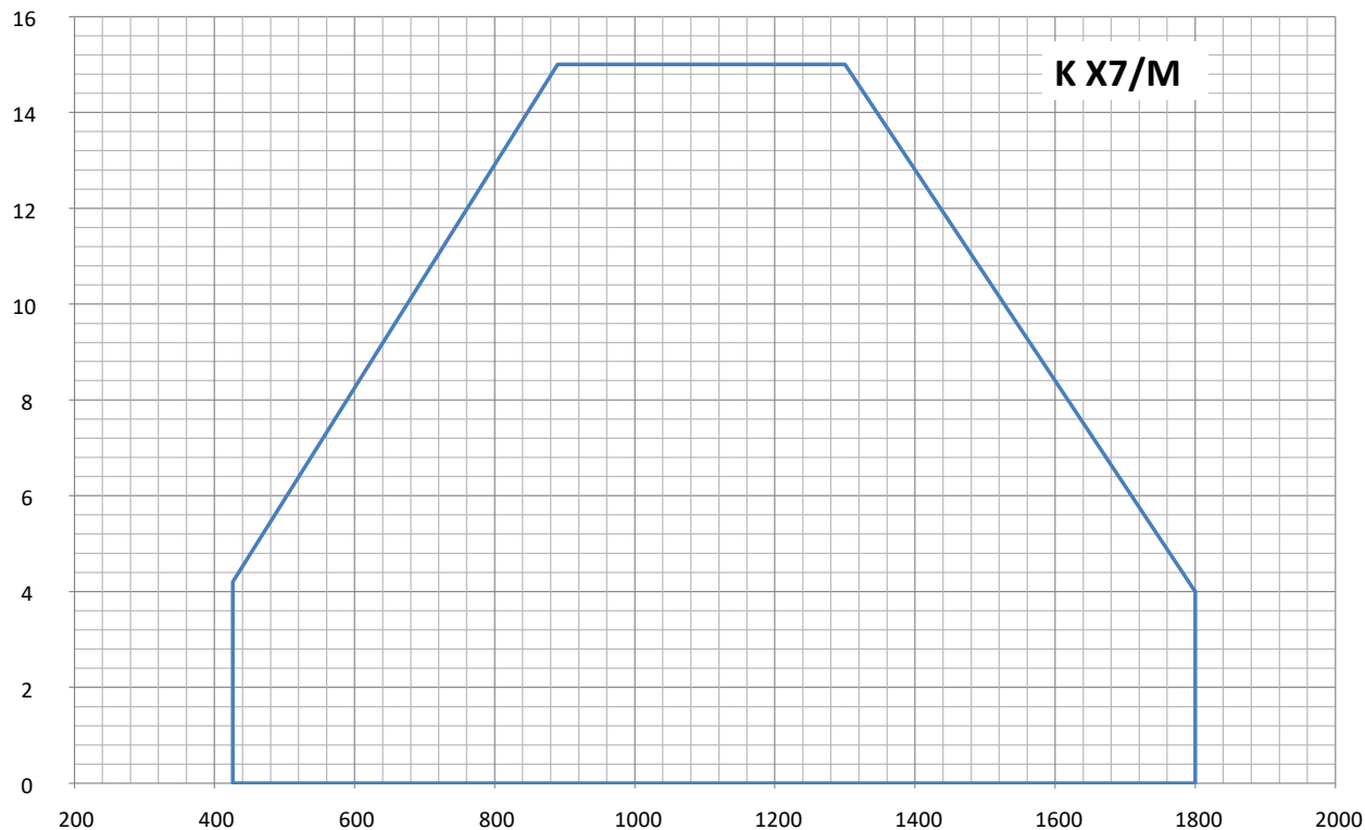
Fig. X = Potenza termica [kW] Y = Pressione in camera di combustione [mbar]
