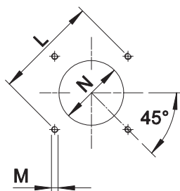
Fig. Flangia fissaggio bruciatore
