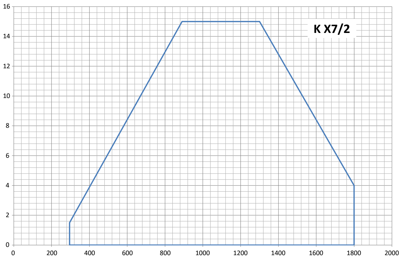
Fig. X = Potenza termica [kW] Y = Pressione in camera di combustione [mbar]
