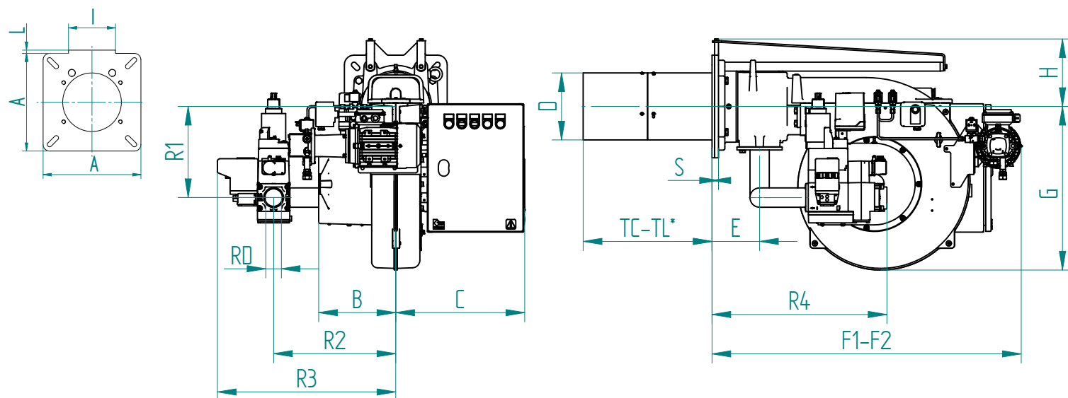
Fig. Dimensioni ingombro: K X6/2 EVO - K X7/2
