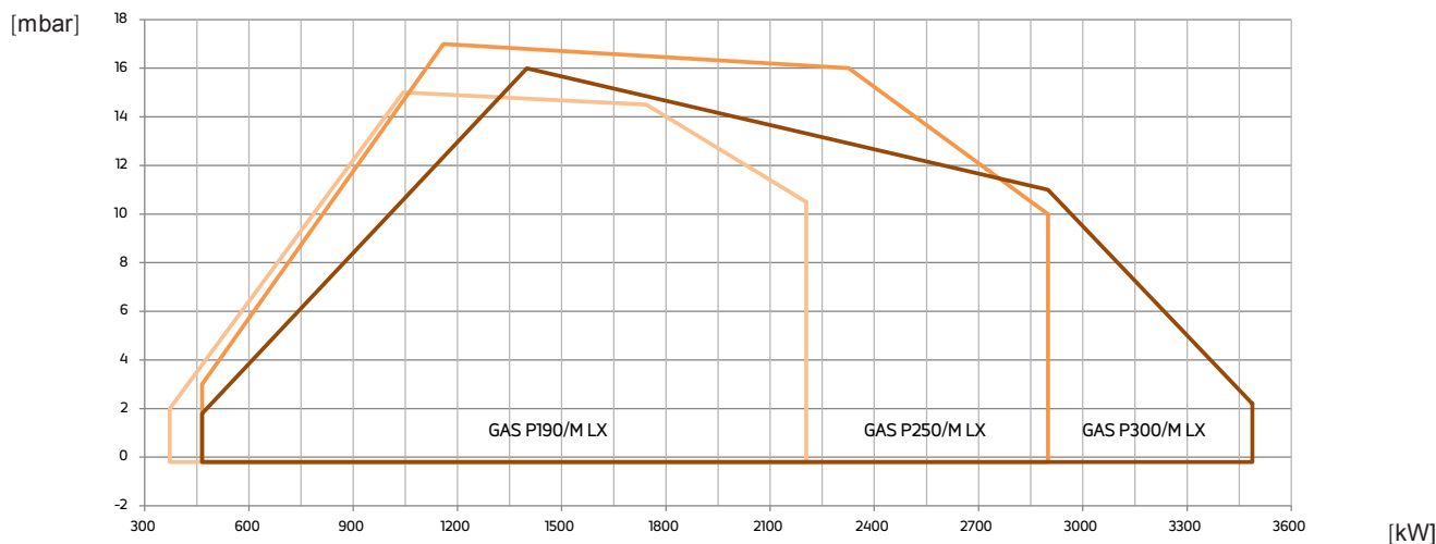
Fig. 3 X = Potenza termica Y = Pressione in camera di combustione
