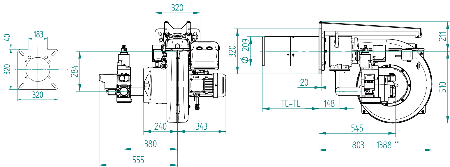
Fig. Dimensioni GAS P130/2CE EVO
