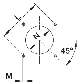
Fig. 4 Фланец для установки горелки
