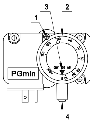
Fig. 8 MOD. DUNGS: 1-Винт-заглушка 2-Регулировочная гайка
