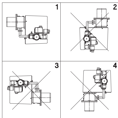
Fig. 3 положение горелки
