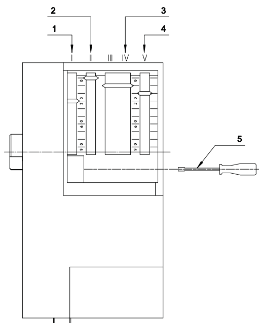
Fig. 9 SIEMENS SQN91.140...
