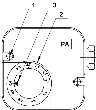
Fig. 7 1-Винт заглушка 2-Регулировочная гайка 3-Указатель регулировки
