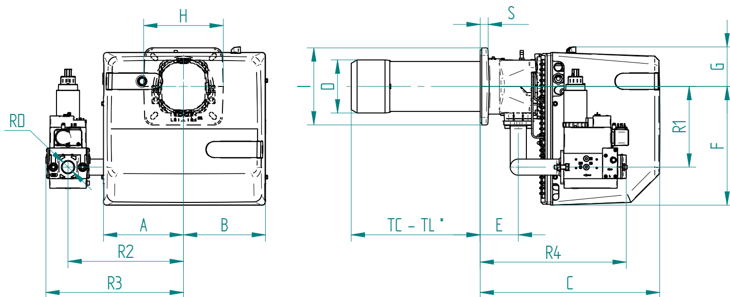
Fig.2 Размеры
