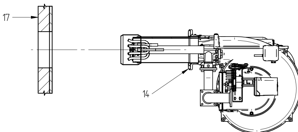
Fig. 4 СХЕМА УСТАНОВКИ ГОРЕЛКИ GAS XP60/MCE-EVO
