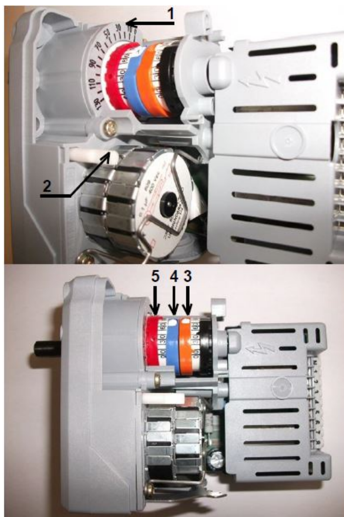
Fig. 15 SIEMENS SQN71.424A20
