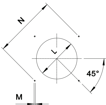
Fig. 6 Фланец для установки горелки
