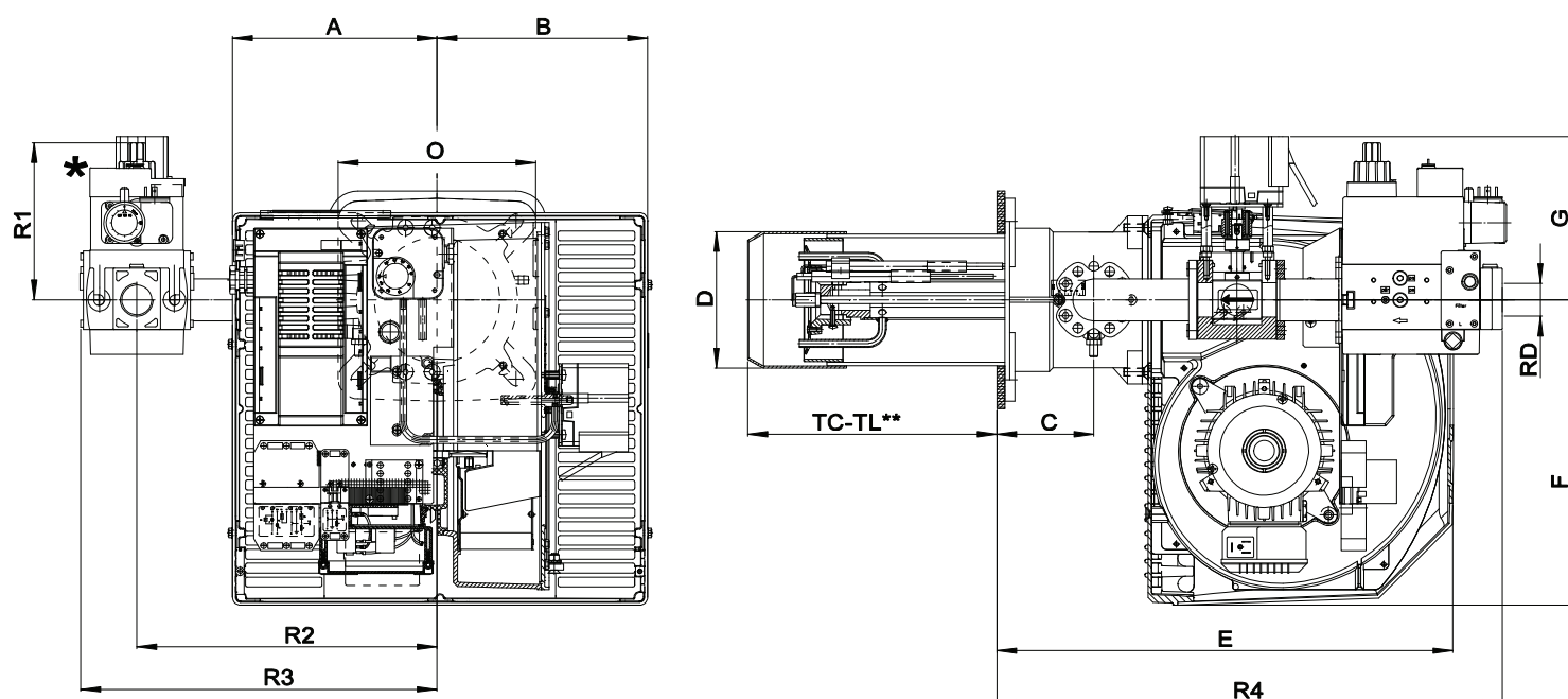
Fig. 3 РАЗМЕРЫ
