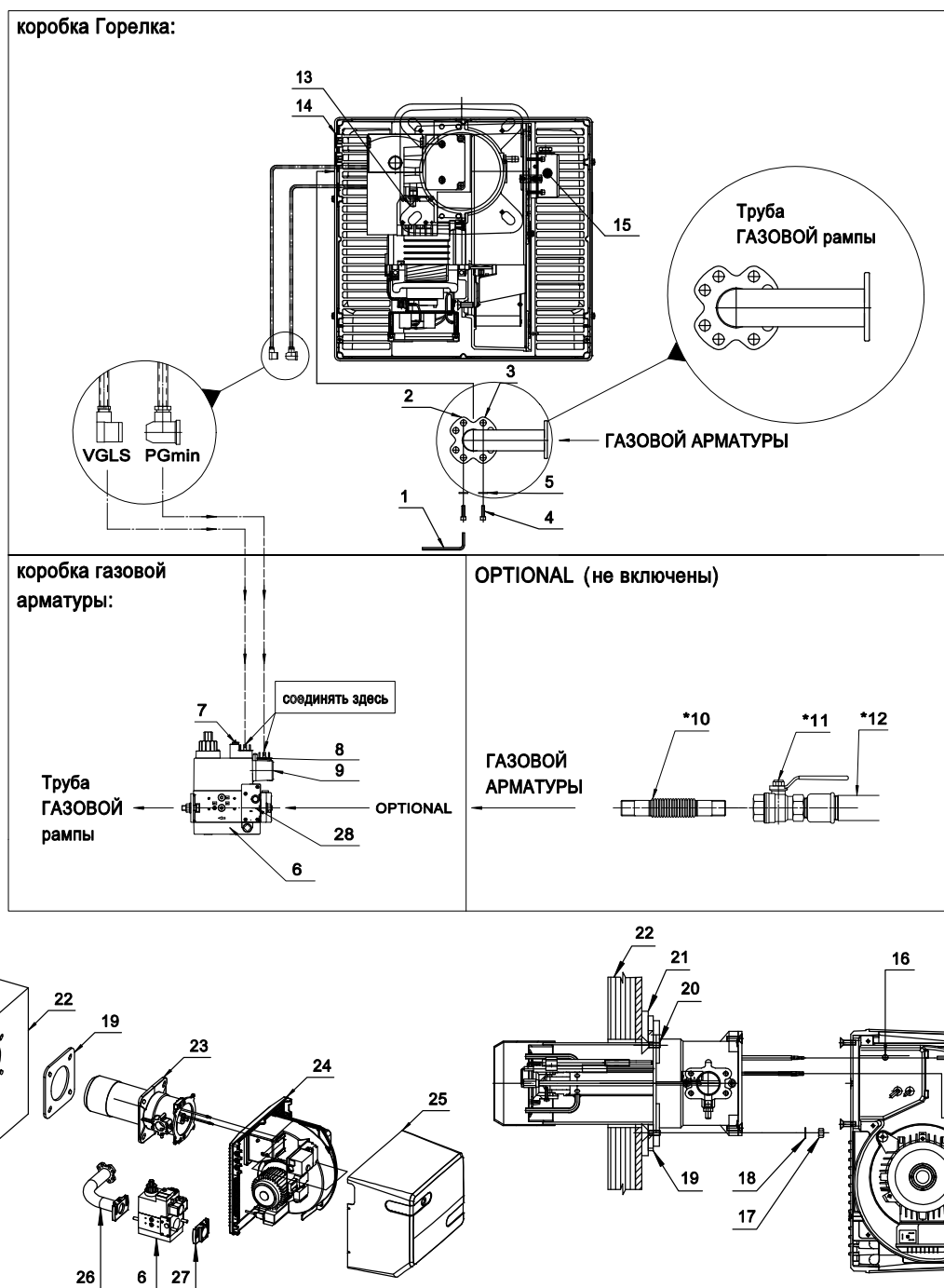
Fig. 7 СХЕМА УСТАНОВКИ ГОРЕЛКИ GAS X5CE
