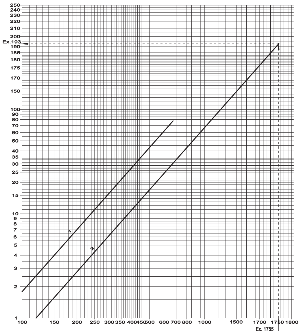
Fig. 23 Ось X= РАСХОД ГАЗ [м3/час] ; Ось Y= PD: давление график [мбар]
