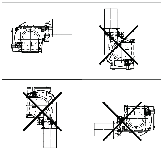
Fig. 7 ПРАВИЛЬНОЕ РАСПОЛОЖЕНИЕ ГОРЕЛКИ
