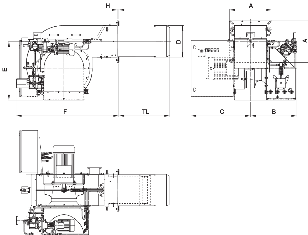
Fig. 2 Burner dimensions
