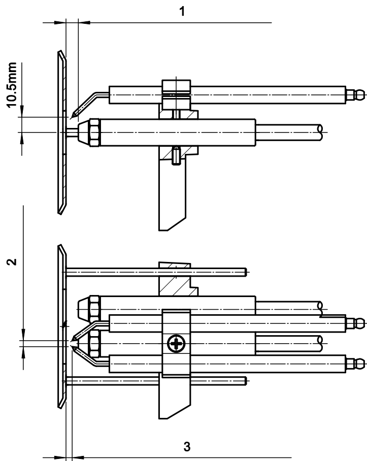
Fig. 13 УСТАНОВКА ЭЛЕКТРОДОВ
