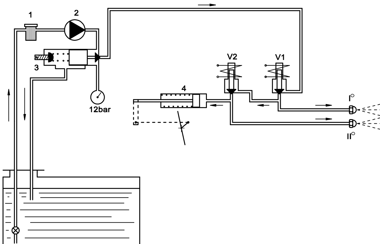
Fig. 9 ГИДРАВЛИЧЕСКАЯ СХЕМА
