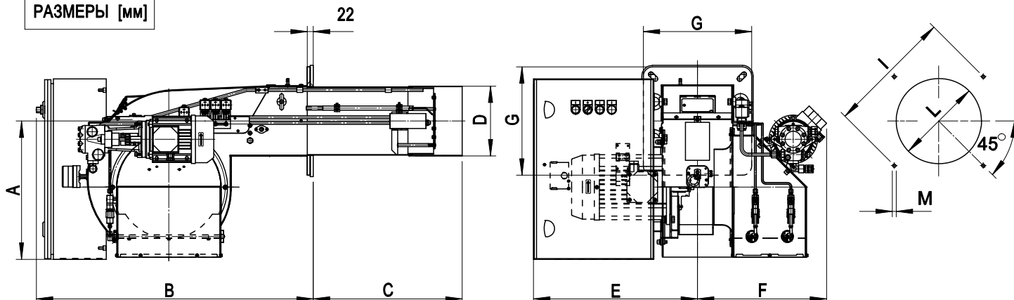
РАЗМЕРЫ [мм]
